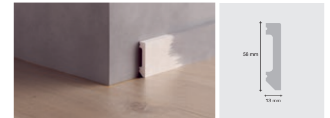
Vannbestandig og malbar sokkellist PGHSK58PAINT, 2400 x 13 x 58 mm
