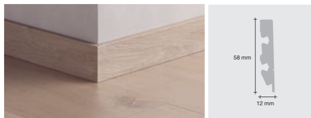
Fargematchet sokkellist PGSK(-), 2400 x 12 x 58 mm*
